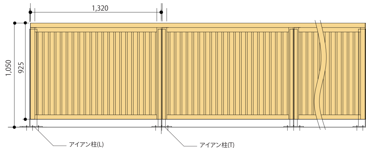
【木塀 参考図】 木塀パネル:W1320×H925
